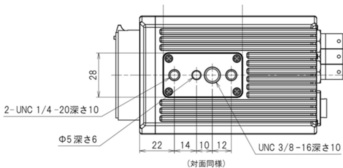
ボックスカメラ底面図
