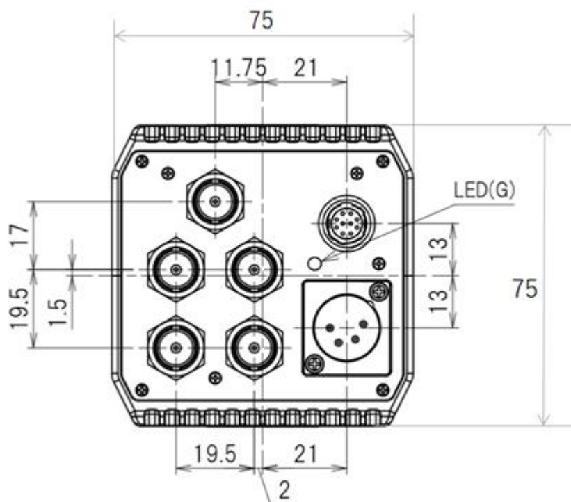
ボックスカメラ背面図
