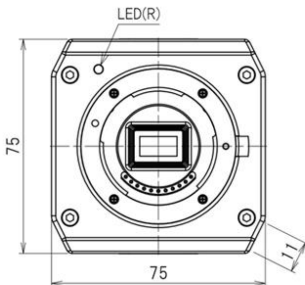
ボックスカメラ前面図
