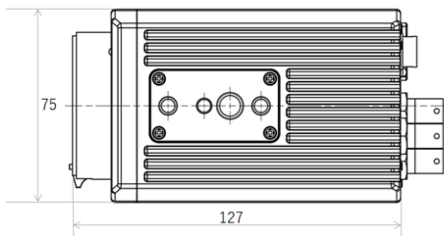
ボックスカメラ天面図
